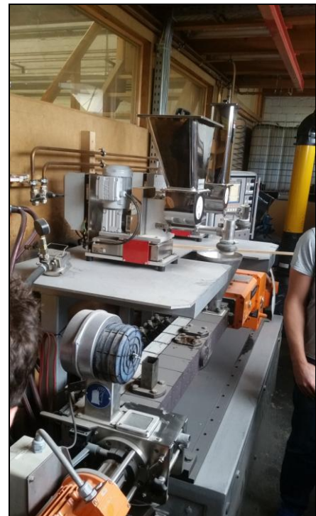
Φωτ. από την επίδειξη παραγωγής WPC που μας έγινε στο pilot plant ( extruder )
