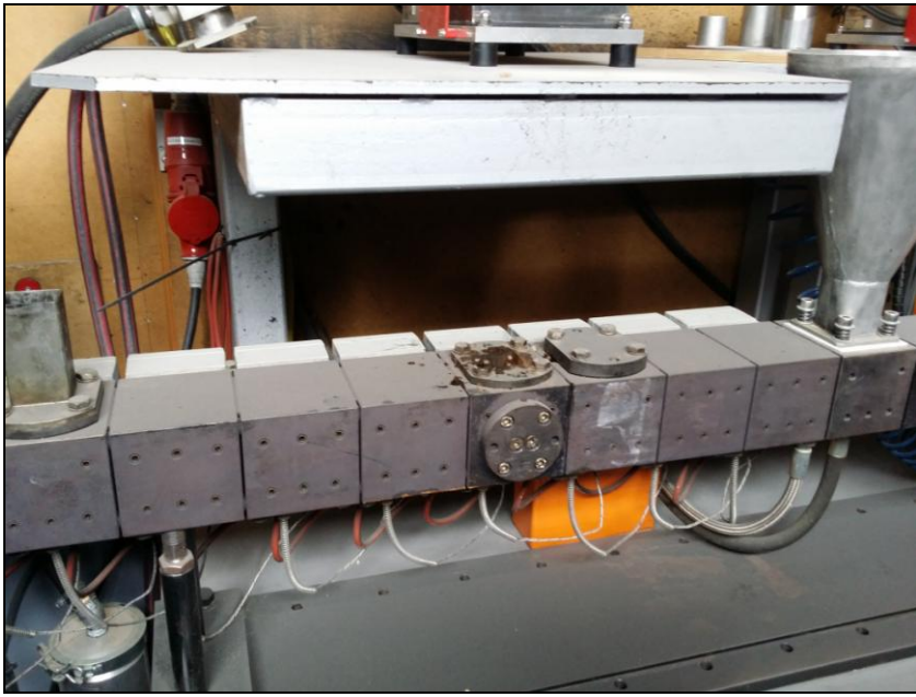
Φωτ. από την επίδειξη παραγωγής WPC που μας έγινε στο pilot plant ( extruder )
